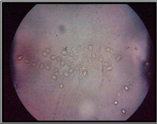
Figure 22: Oocystes d' E. tenella
