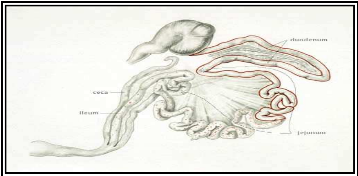
Figure 15 : localisation d' Eimeria brunetti dans l'intestin (Dr. Constantinescu. G.)
