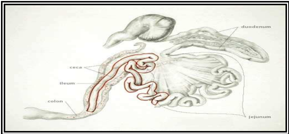
Figure 19 : La localisation d' Eimeria mitis dans l'intestin (Dr. Constantinescu. G.)
