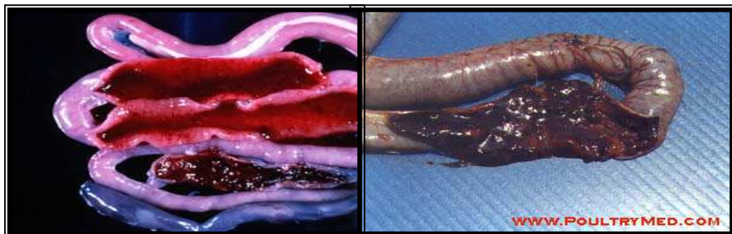
Figure 12 : muqueuse oedémateuse et recouverte d'un exsudat associée à des lésions hémorragiques dans le petit intestin.
