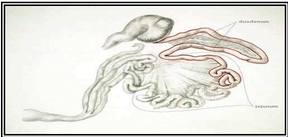
Figure 20 : La localisation d' Eimeria preacox dans l'intestin (Dr. Constantinescu G.).
