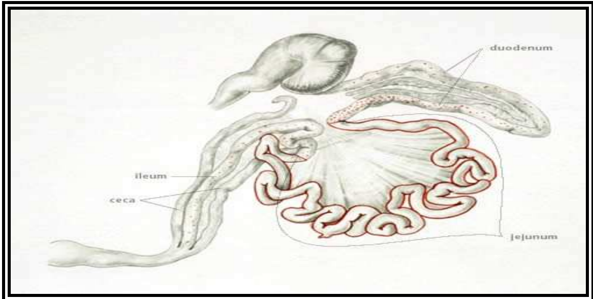
Figure 13 : La localisation d' Eimeria maxima dans l'intestin (Dr. Constantinescu G.).
